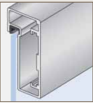
PROFIL D
