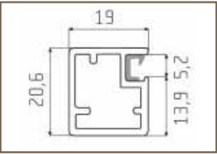
PROFIL H
