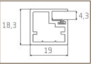
PROFIL I
