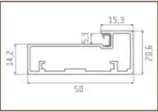
PROFIL M
