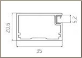
PROFIL N
