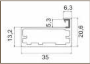
PROFIL K
