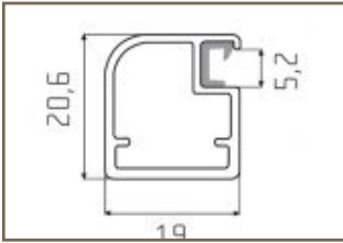
PROFIL J
